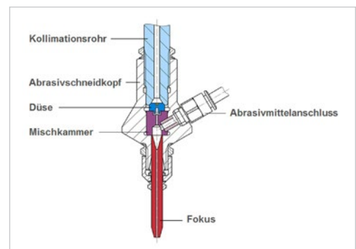
Abrasivkopf
